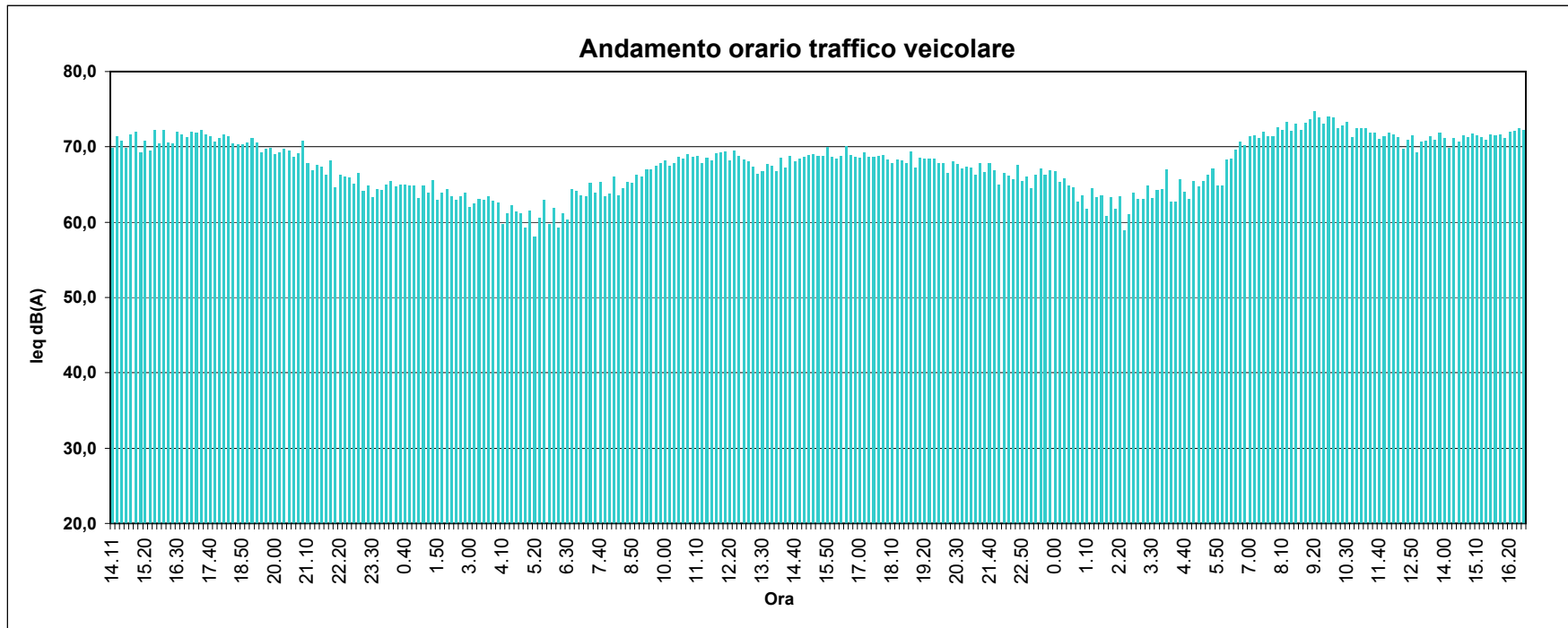
RAPPRESENTAZIONE GRAFICA ANDAMENTO ORARIO DEL TRAFFICO VEICOLARE (LEQ dBA - LIV. STATISTICO LN 95)
