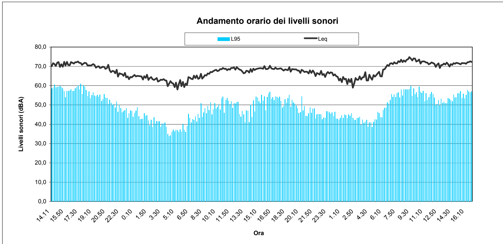
RAPPRESENTAZIONE GRAFICA ANDAMENTO ORARIO DEL LIVELLO EQUIVALENTE (Leq, dBA) A CONFRONTO CON LN 95
